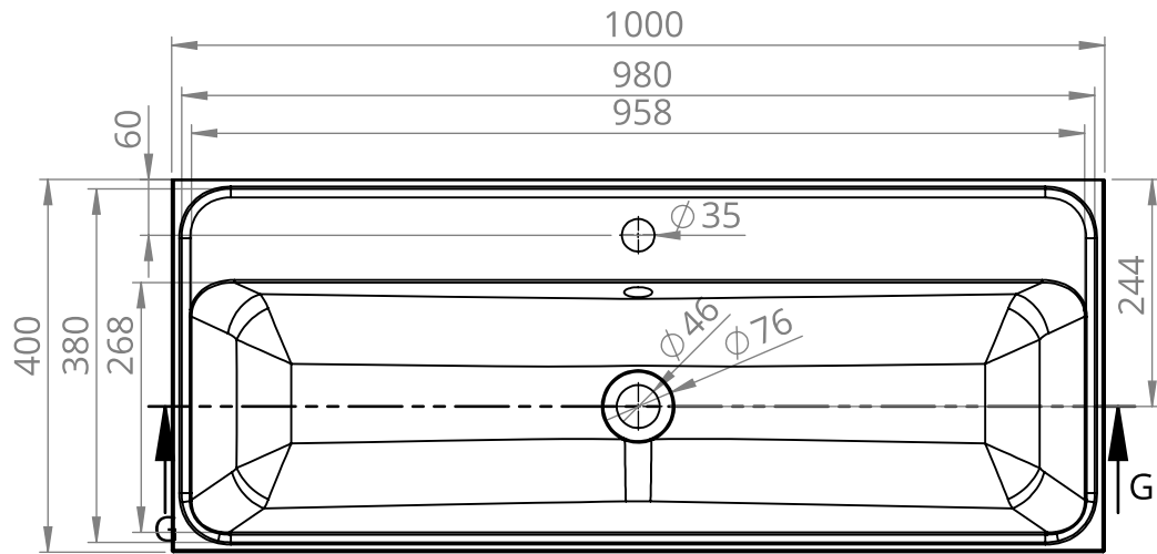
PRZEKRÓJ H-H SKALA 1 : 9
