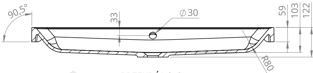
PRZEKRÓJ G-G SKALA 1 : 9
